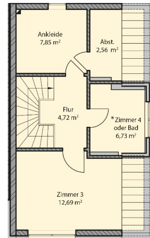
Dachgeschoss
