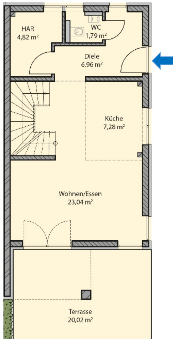
Erdgeschoss
