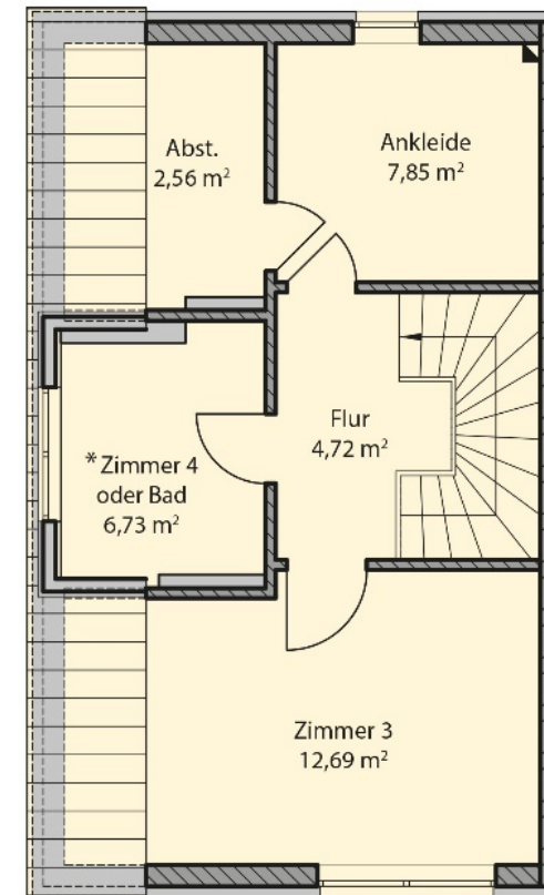
Dachgeschoss
