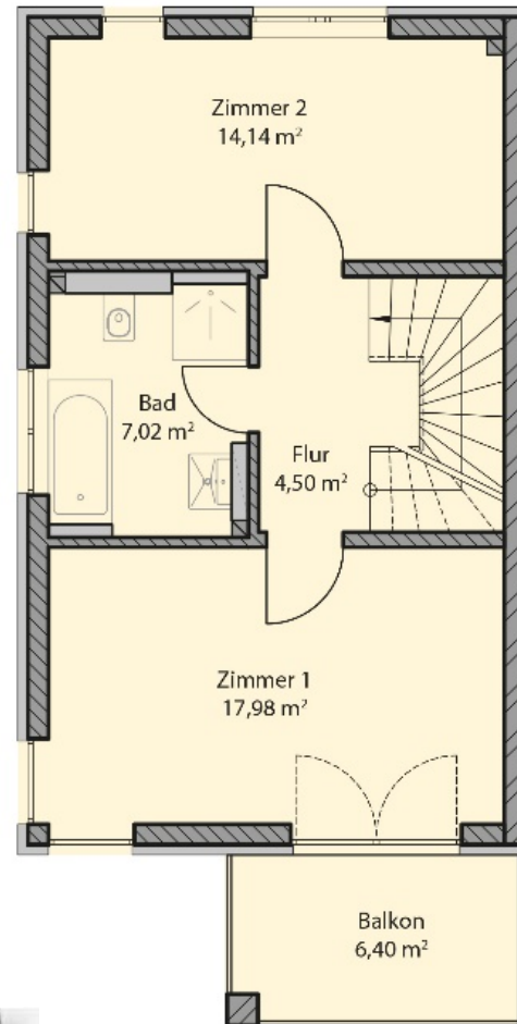
Obergeschoss
